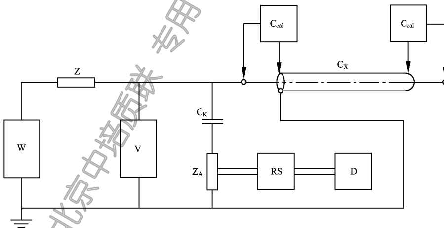
图 4 终端阻抗 Z_W 的连接
