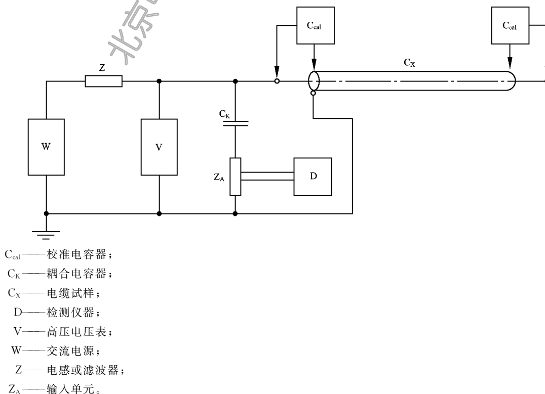
图 1 输入单元 Z_A 与耦合电容器 C_k 串联
