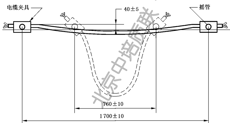
图 3 曲挠试验装置
