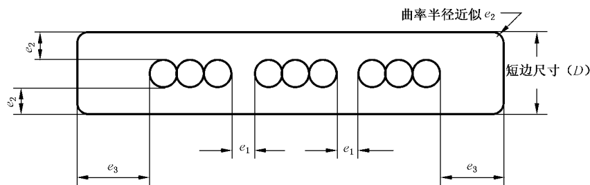
图 1 电缆断面图
