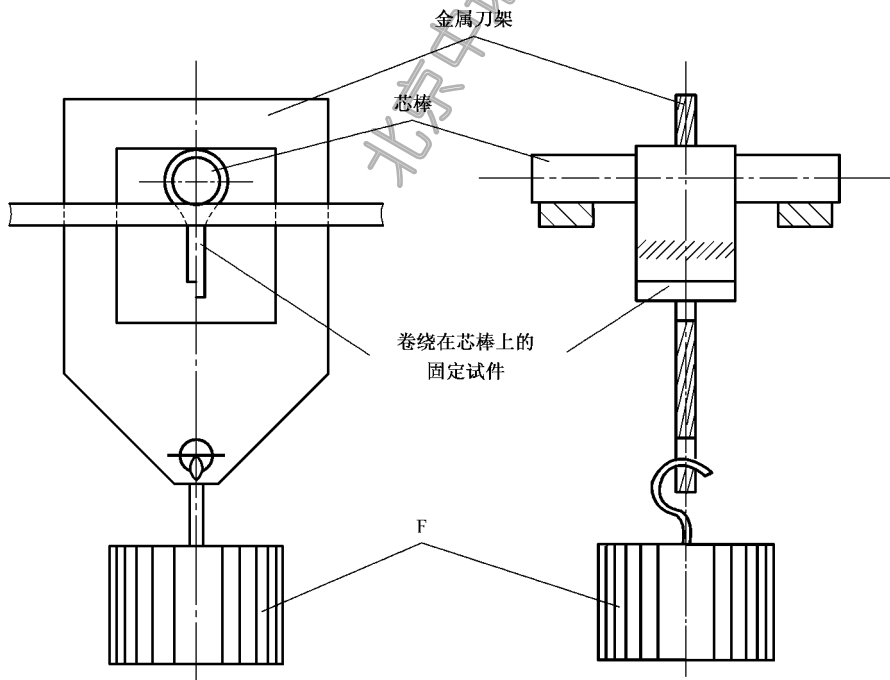
图 2 压痕试验装置
