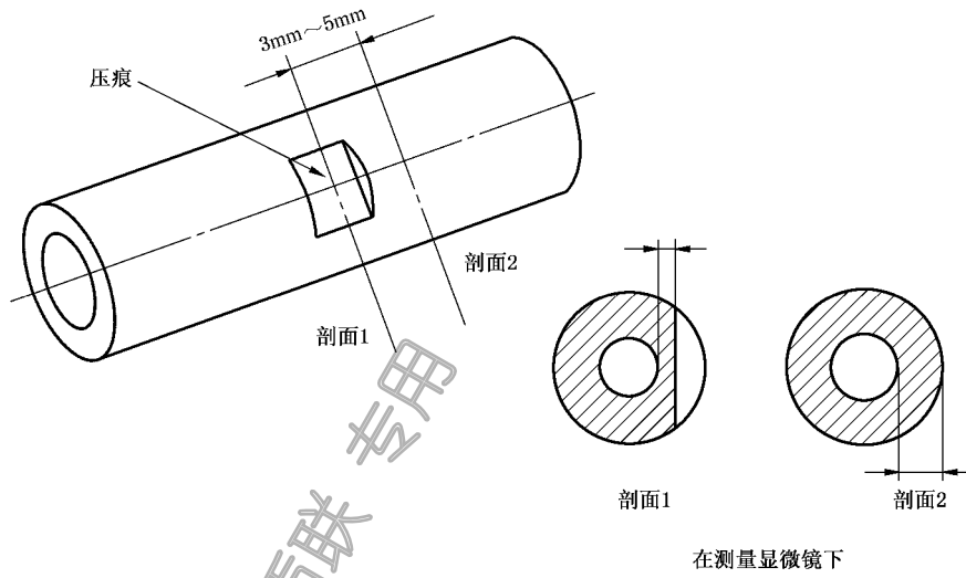
图 3 小试样的压痕测量
