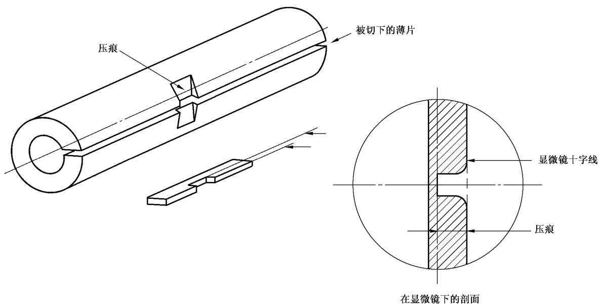
图 2 压痕测量
