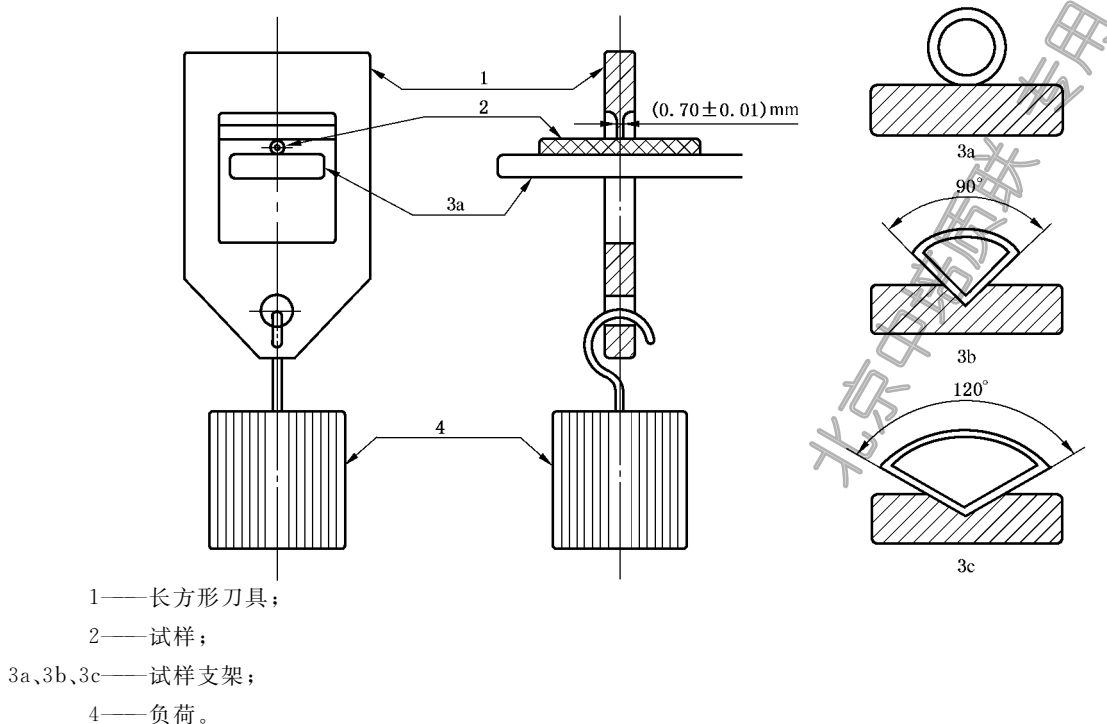
图 1 压痕装置
