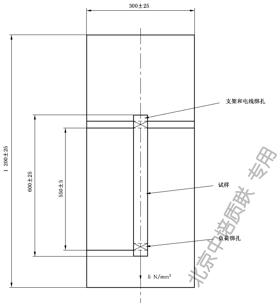
图 1 试样放置(金属导体)
