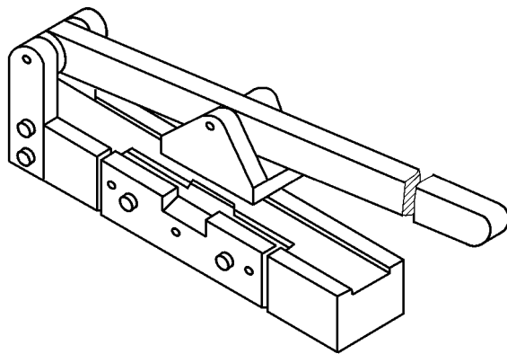
图 1 刻痕装置
