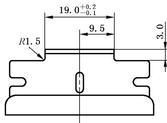
图2 刀片
