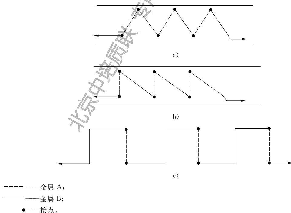
图 3 热电堆设计示意图
