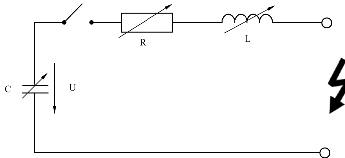
图 F.2 雷电流发生器原理图
