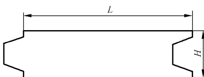
图 3 TG 型产品（榫槽）
