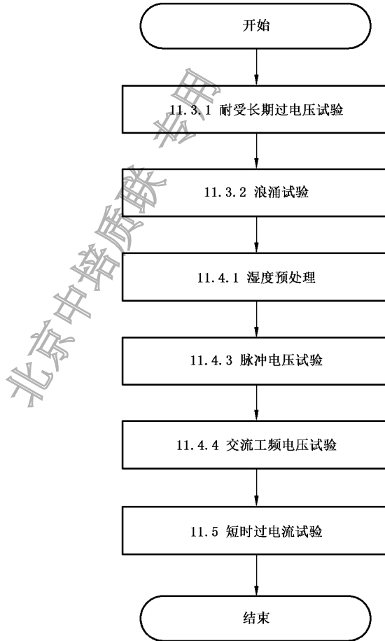
图 A.1 与安全有关的电气试验流程
