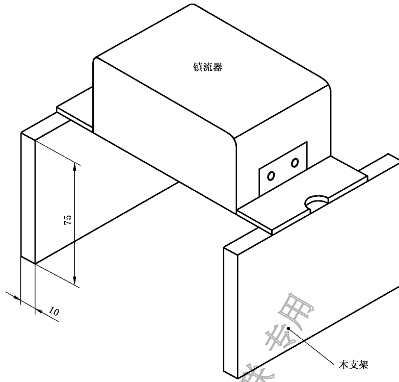
图 H.1 加热试验样品配置图
