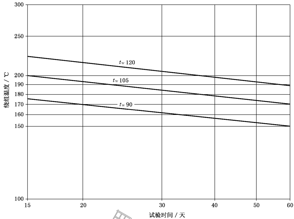
注: 这些曲线仅供参考,并说明常数 S 为 4.500 的公式(2)(见附录 E)
