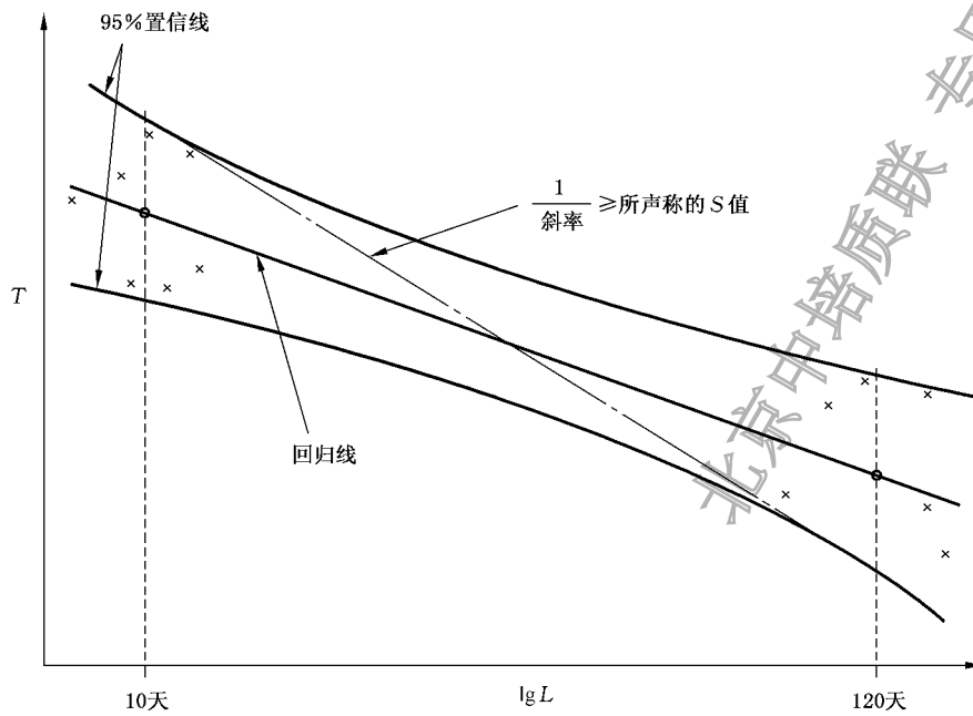
图 E.1 对所声称的 S 值的鉴定
