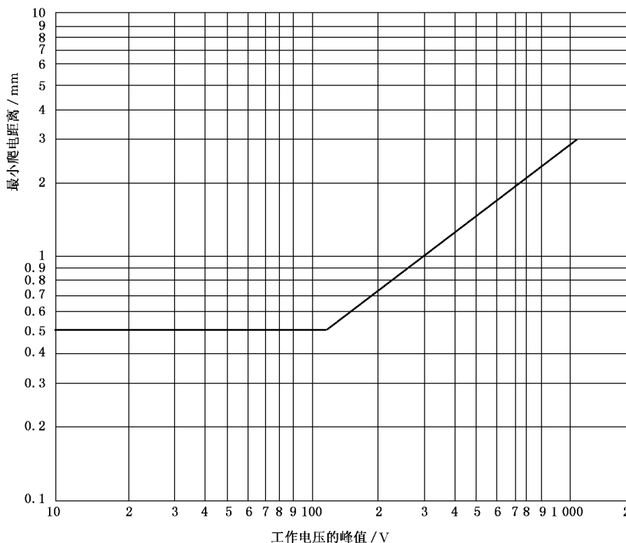
图 2 不与电源连接的印刷电路板上导体之间的爬电距离
