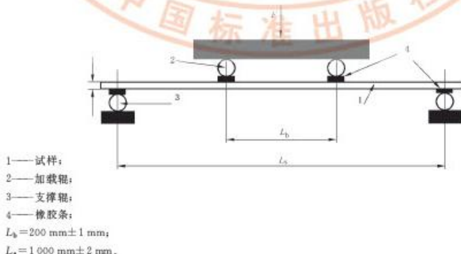
图 B.1 四点弯曲强度试验
