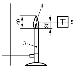
c) 燃烧喷嘴示意图
