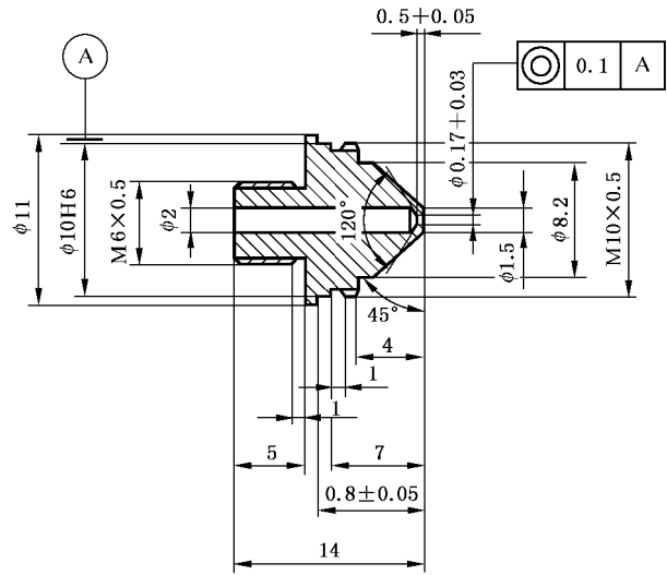
b) 燃气喷嘴
