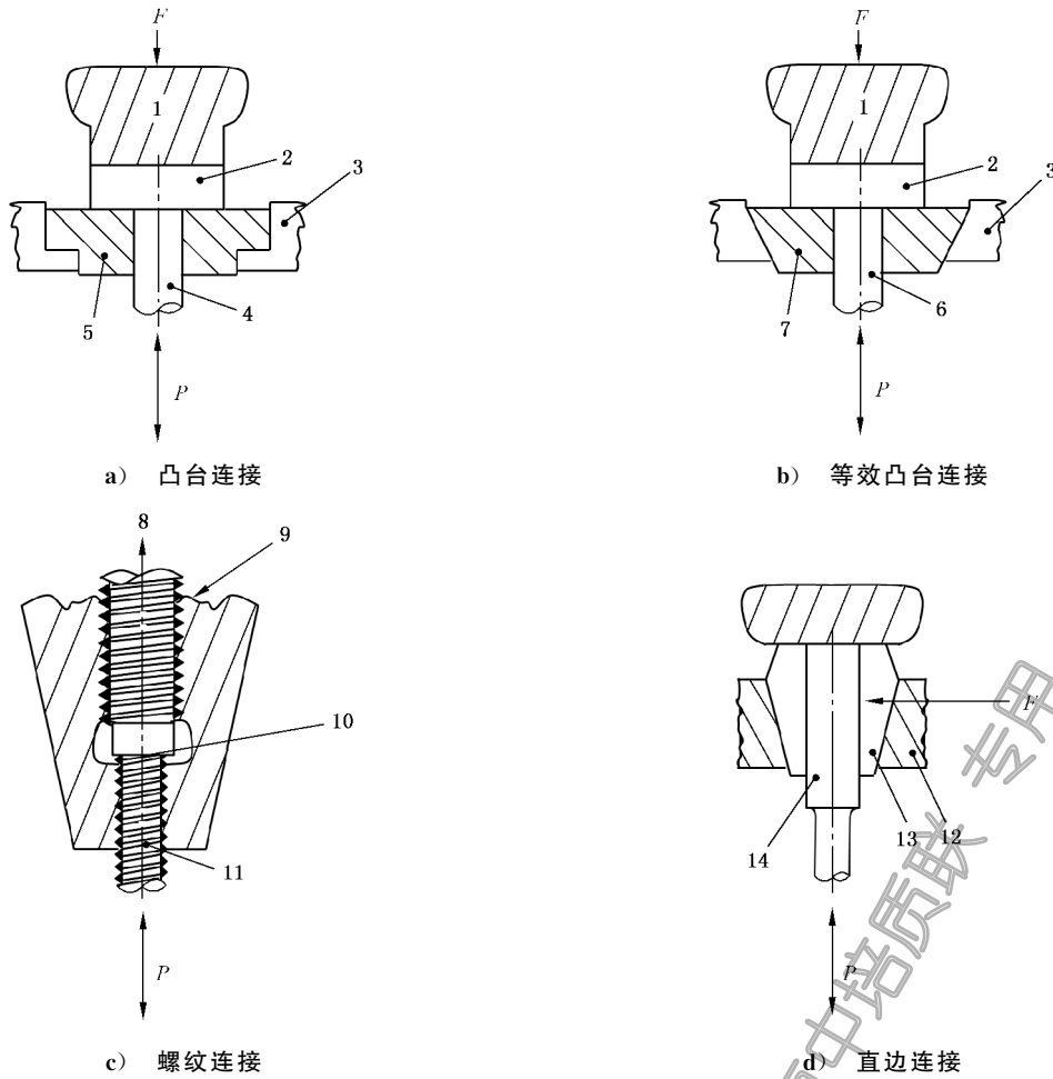
图 5 推荐的蠕变-疲劳试样夹持端示意图
