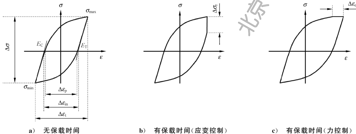
图 1 应力-应变滞后迴线示意图
