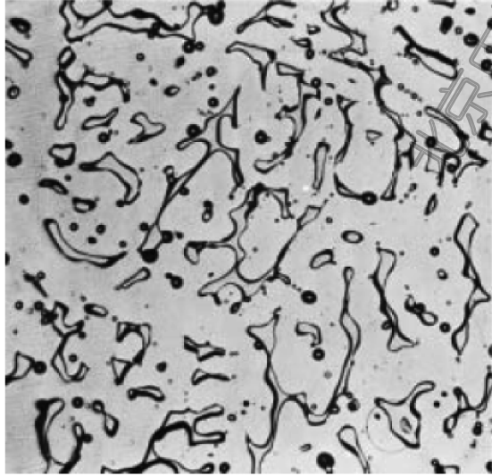
图 11 游离铁素体组织(四类)250×
