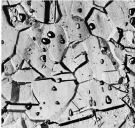
图 8 阶梯组织(一类)500×
