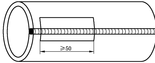
图 1 焊管舟形试样取样
