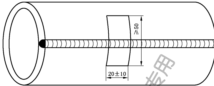
图 2 焊管弧形试样取样
