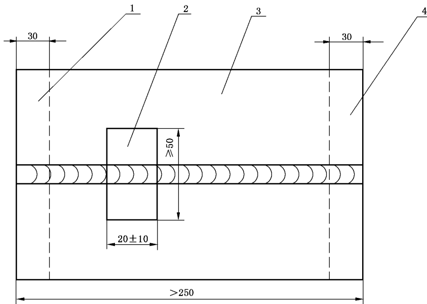
图 4 堆焊焊条试样取样
