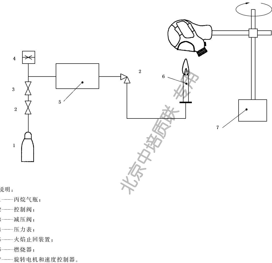
图 7 可燃性检测装置示意图
