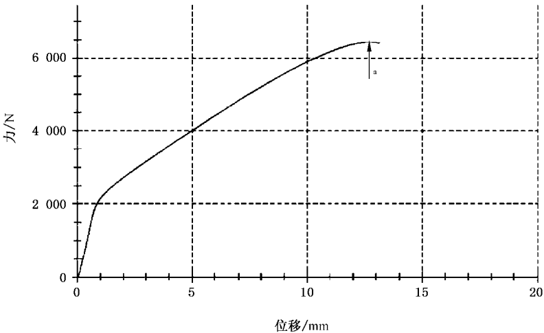
图 A.1 弯曲试验压头力-位移曲线
