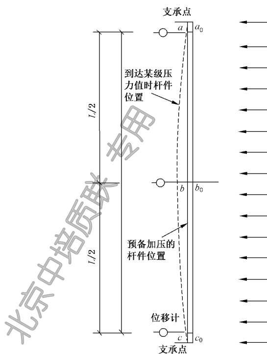
图 6 简支梁型式杆件测点分布示意图
