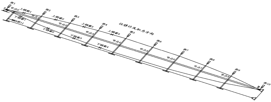
图 C.5 自平衡索杆结构加载及测点分布示意图
