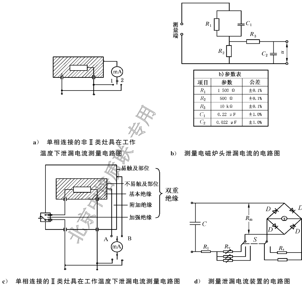
图 14 测量泄漏电流的电路图
