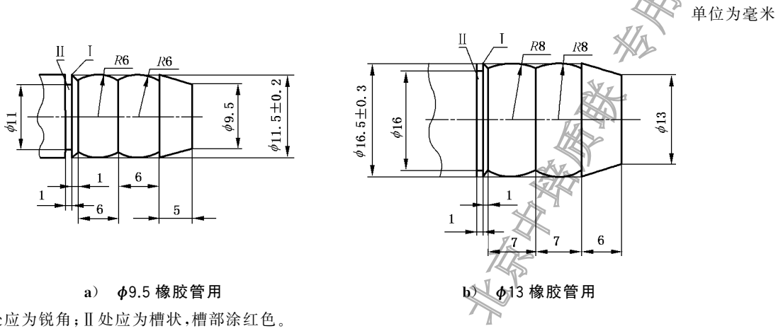
图 2 软管接头的形状及尺寸
