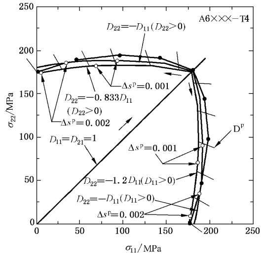
b) 6000 系列铝合金
