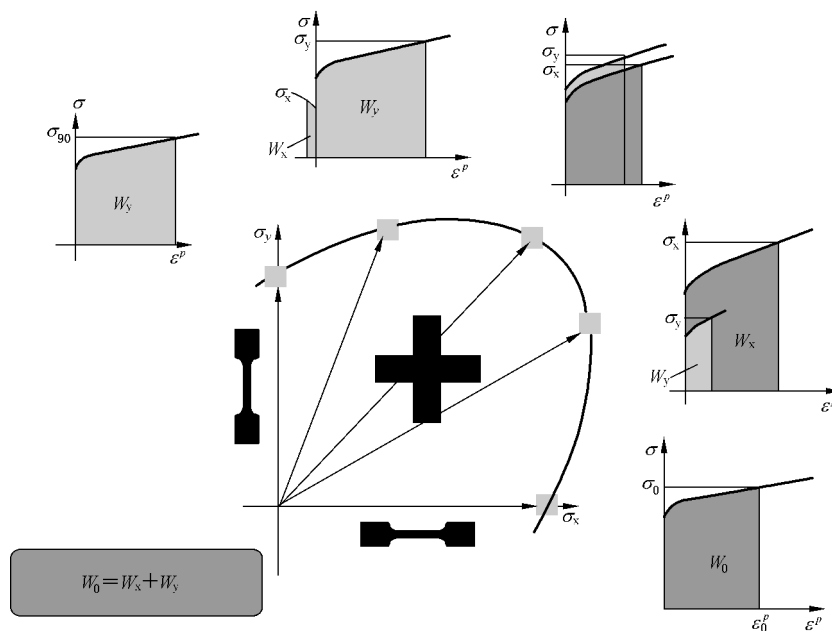
图 D.1 塑性功测定示意图
