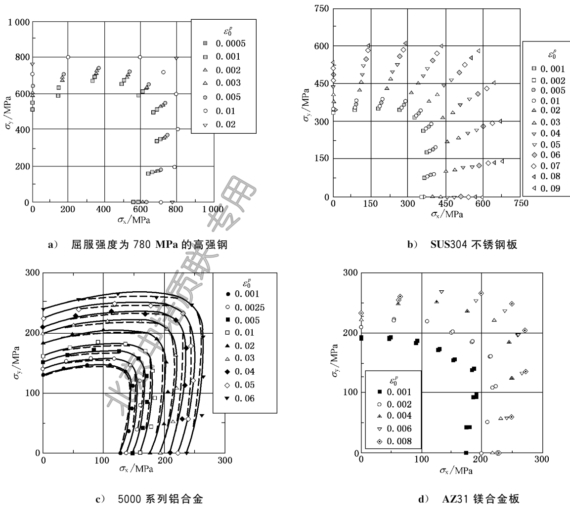
图 D.2 用双向拉伸测试方法测量塑性功的案例
