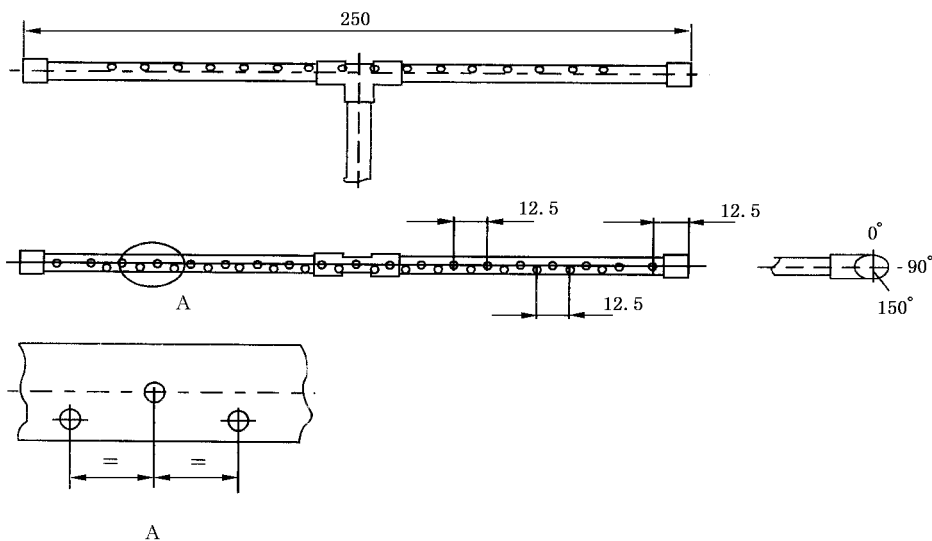
图7 点火器
