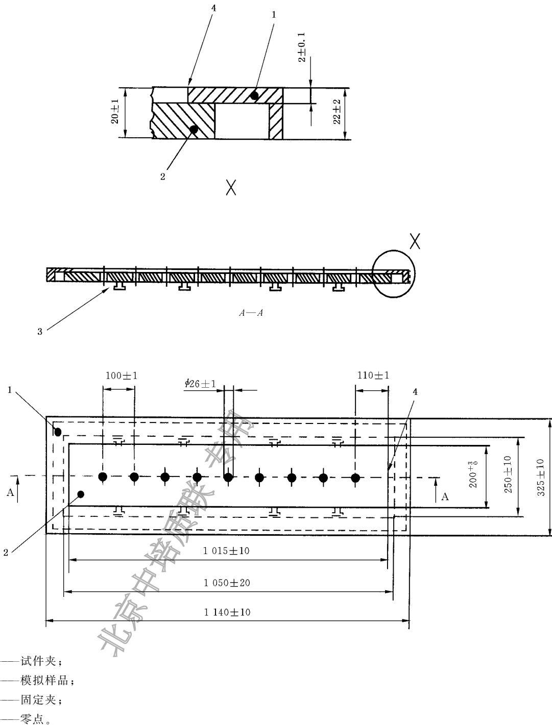
图 6 试件及试件夹具(没有钢尺)
