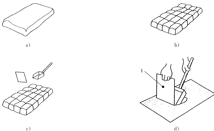
图 4 棋盘缩分法
