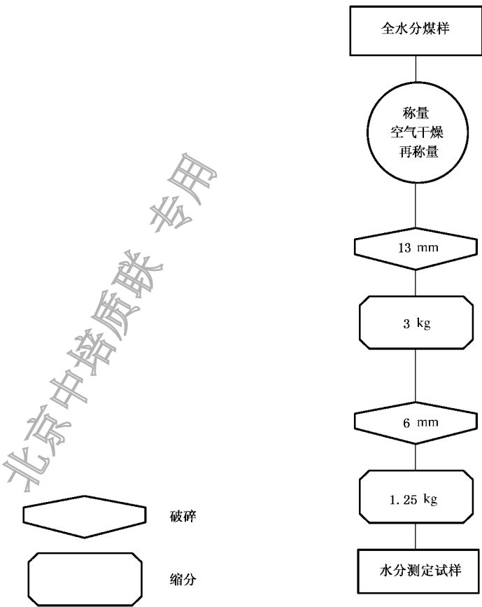
图 8 水分试样两阶段制备程序
