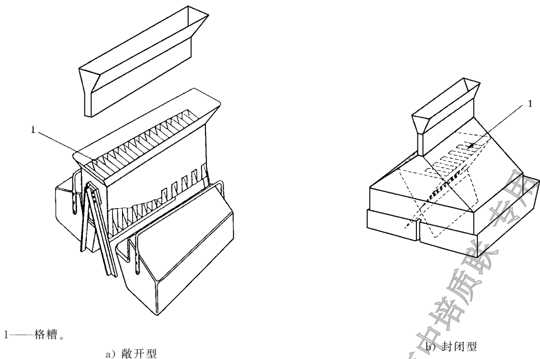
图 3 二分器
