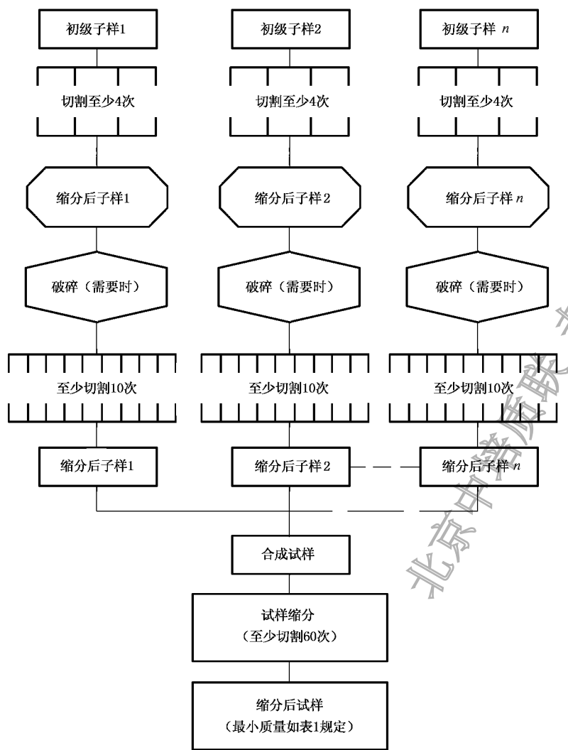
b) 单个子样两阶段缩分 图 2 (续)
