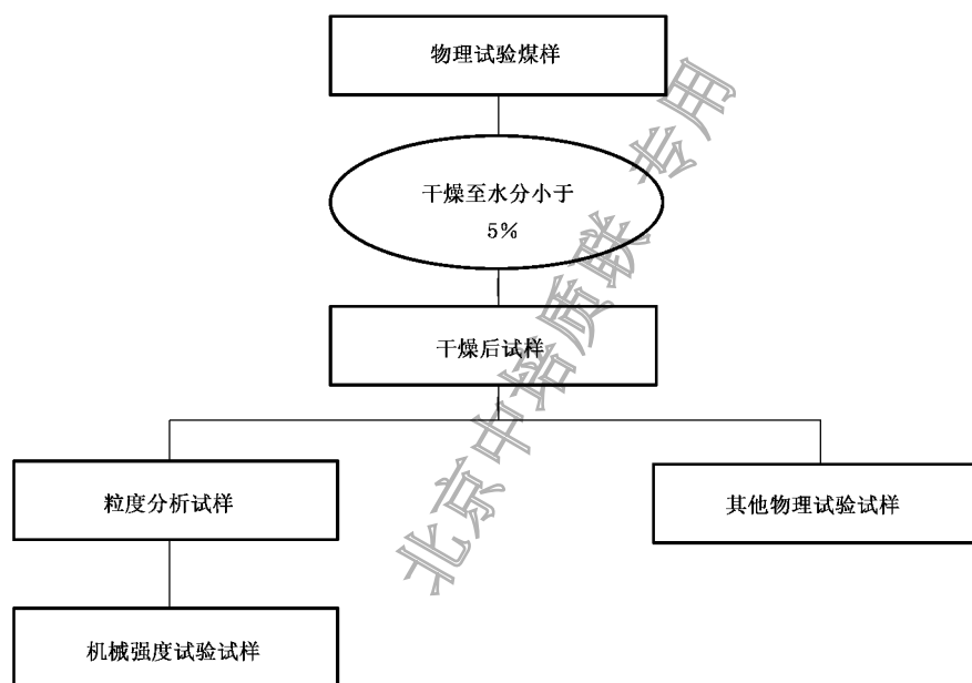
图 11 粒度分析和其他试验煤样制备程序
