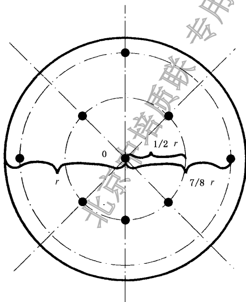
图 7 九点取样法
