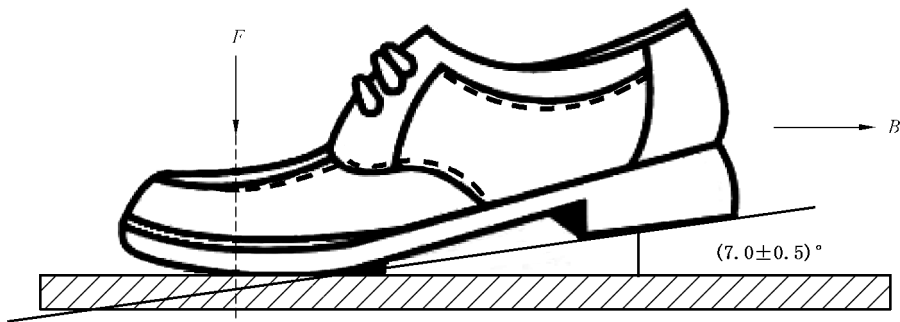
b) 前掌向后滑动
