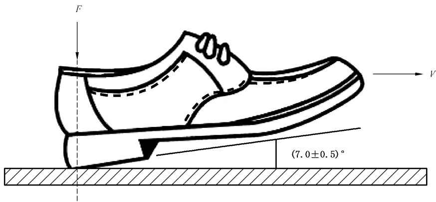
a) 后跟向前滑动
