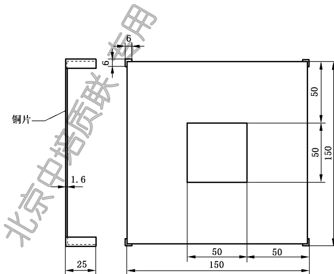
图 A.3 样品支架示意图
