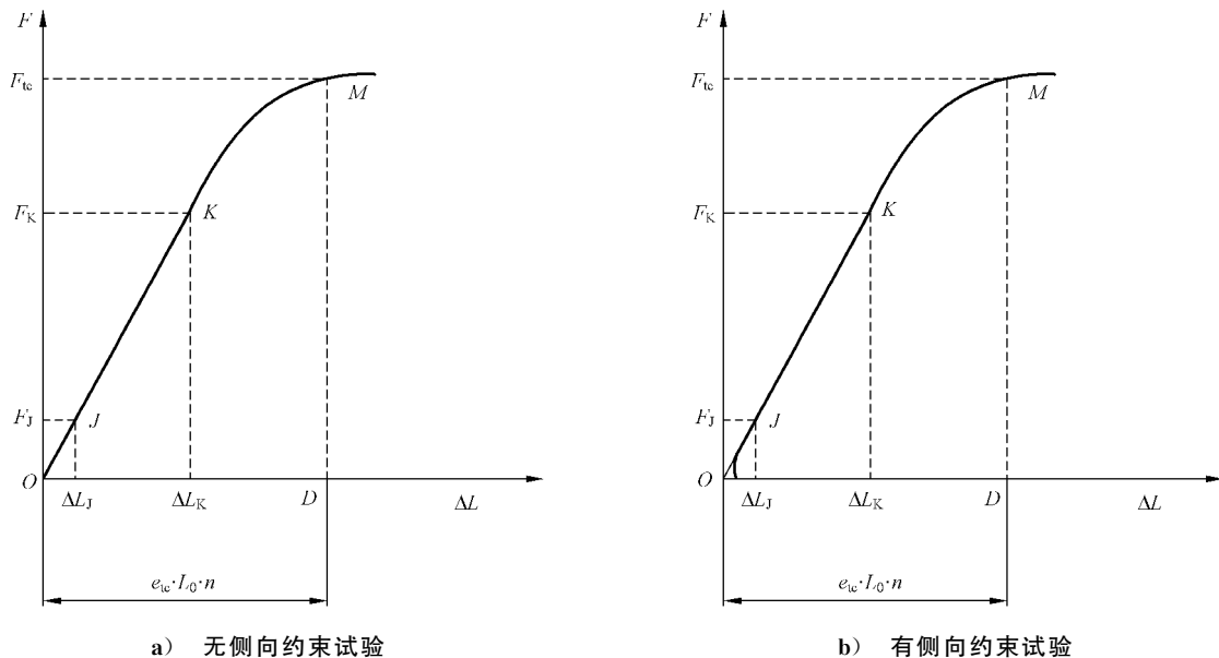
图 11 图解法求 F_{tc}
