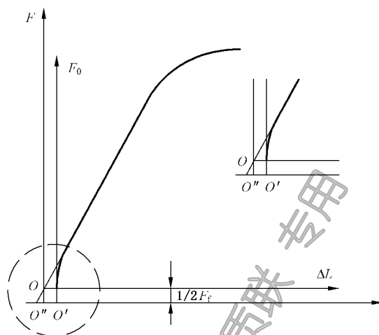
图 8 用图解法确定实际压缩力 F
