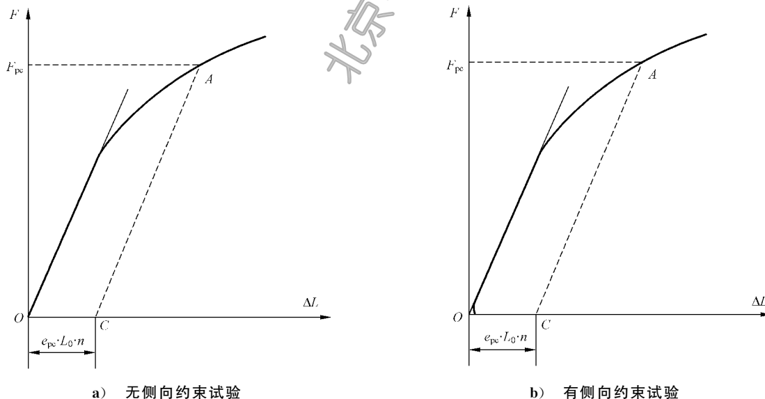
图 9 图解法求 F_{pc}
