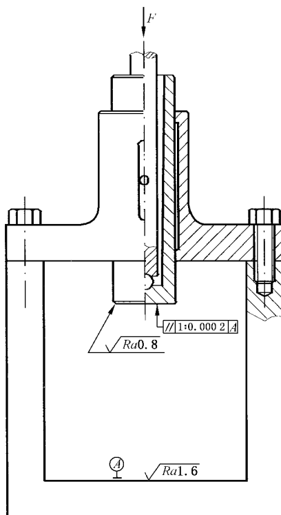
图 5 力导向装置示意图
