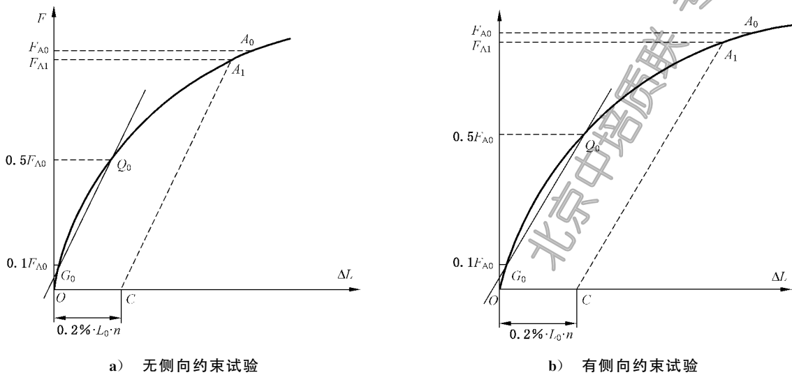
图 10 逐步逼近法求 F_{pc}
