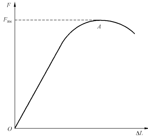
图 13 图解法求 F_{mc}
