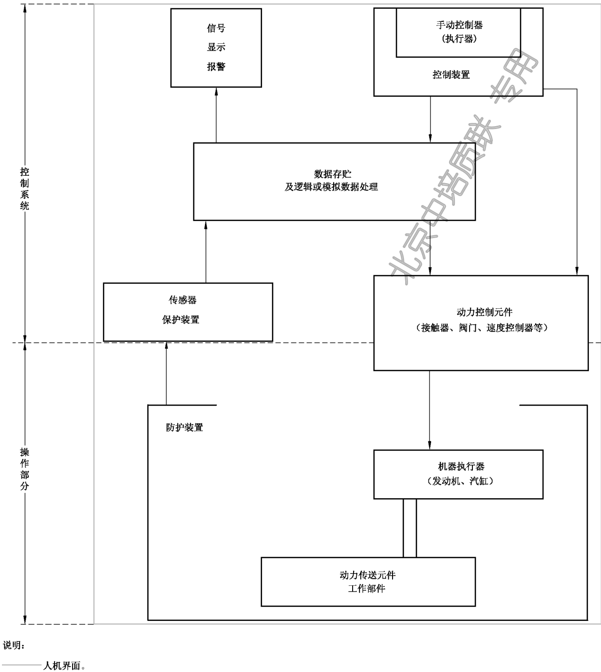
图 A.1 机器的图解表示
