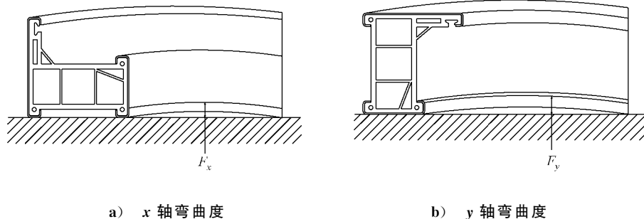
图 A.2 弯曲度测试示意图
