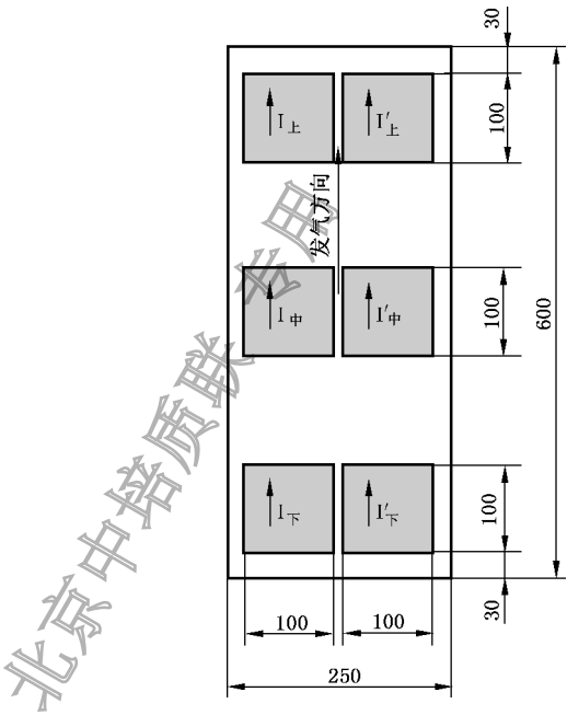
图 3 抗压强度、劈裂抗拉强度试件锯取示意图
