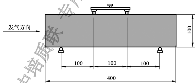
图 7 抗折强度试验示意图
