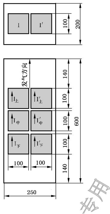
图 12 碳化试件锯取示意图
