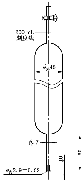
图 5 滴液管
