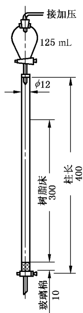
图3 离子交换柱
