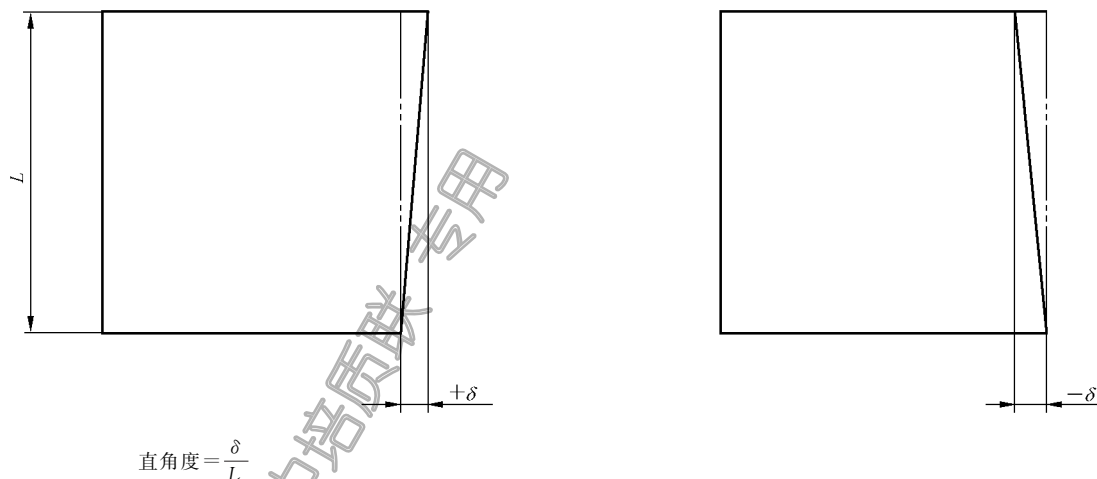
图2 直角度
