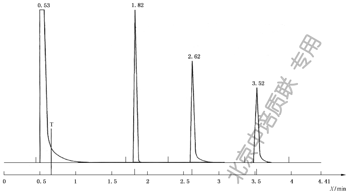
图 1 六亚甲基二异氰酸酯和甲苯二异氰酸酯的气相色谱图
