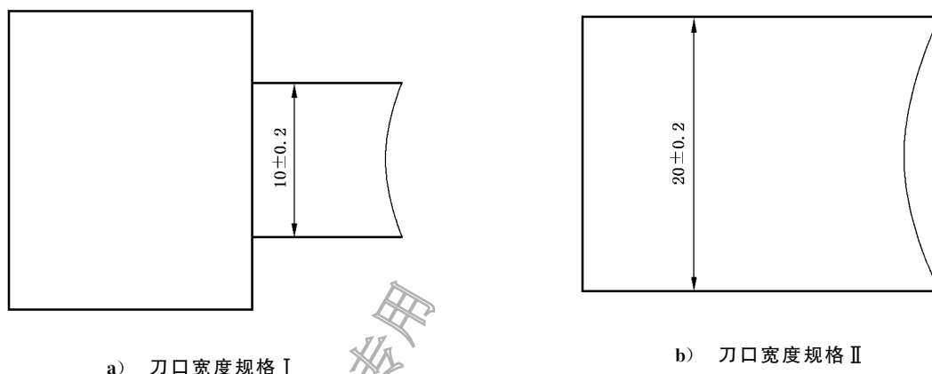
图 1 剥离刀刀口宽度
