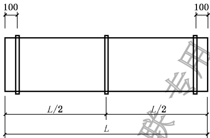
图3 宽度测量位置
