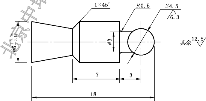
图 9 收缩头
