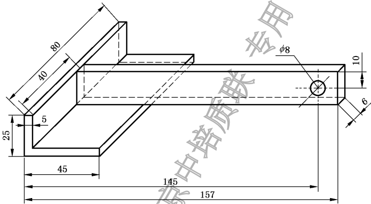
图 10 钢板吊挂件
