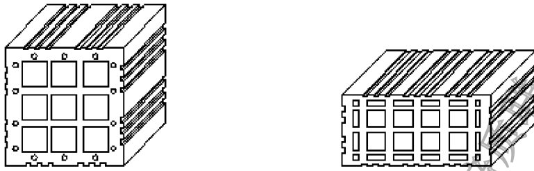
图 B.1 空心砖孔洞排列示意图
