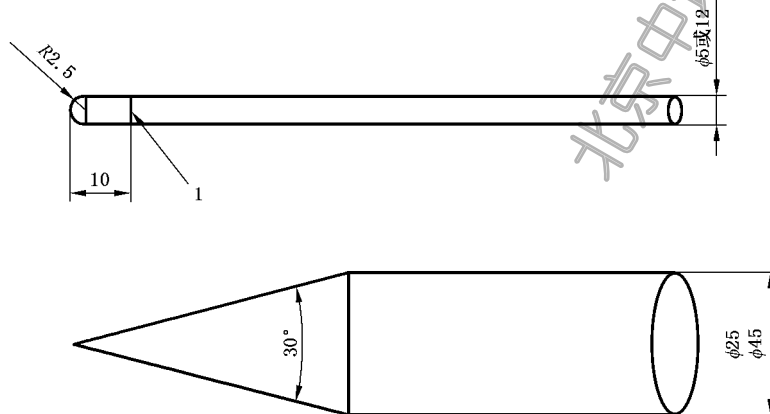
图 6 塞规
