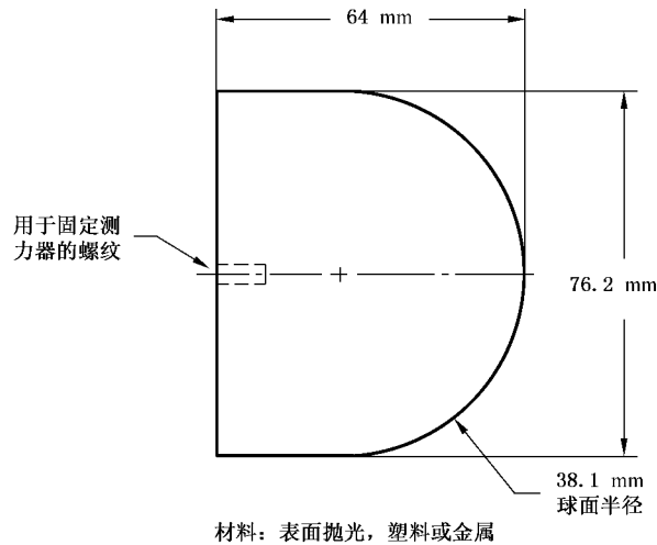
图 21 76.2 mm 塞规
