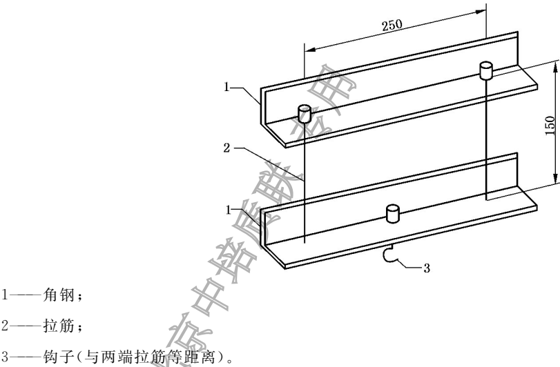
图 13 吊架
