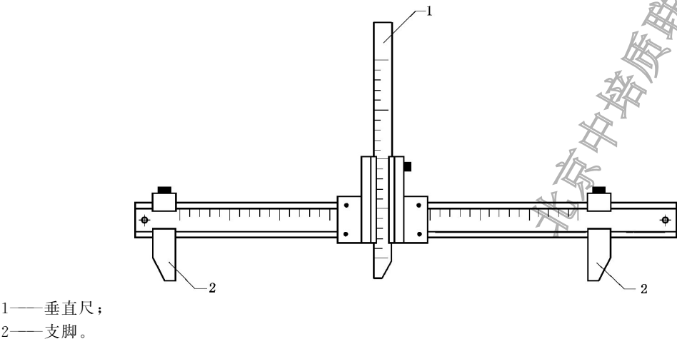
图 1 砖用卡尺
