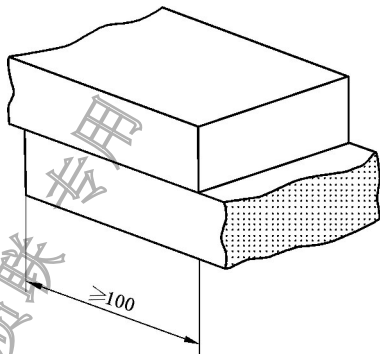
图 12 半砖叠合示意图
