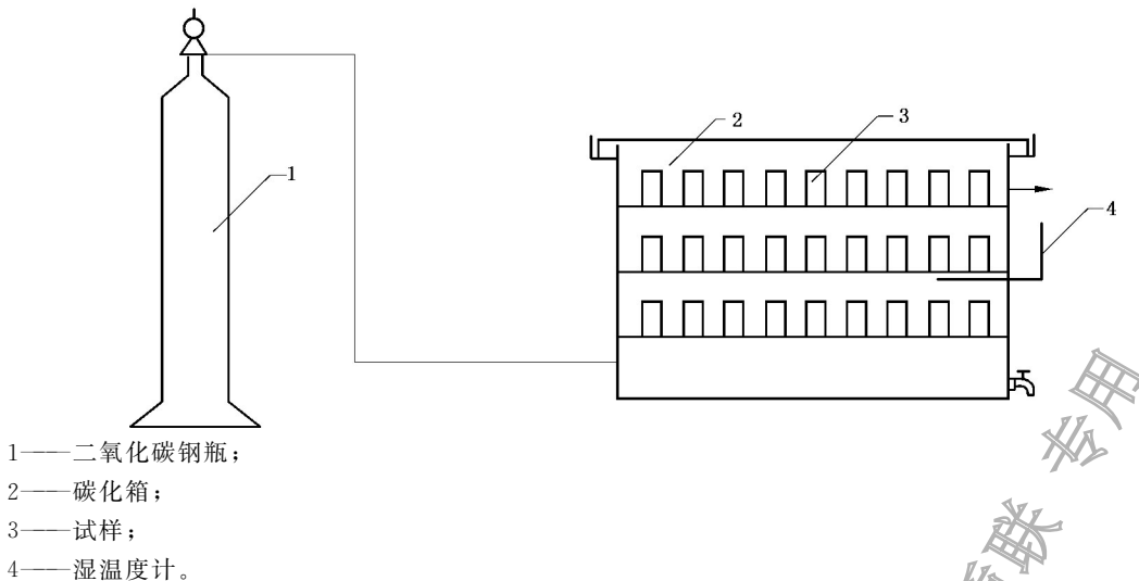
图 16 人工碳化装置示意图
