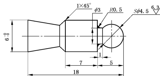
图 15 收缩头
