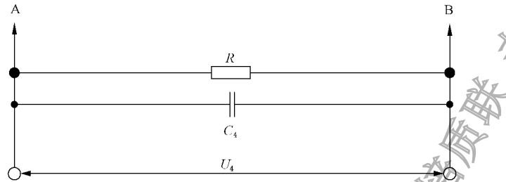
图 G.3 摆脱加权接触电流的测量网络(用于 I 类可移式灯具)
