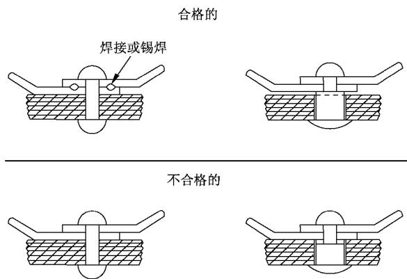
图 16 單式接线端子
