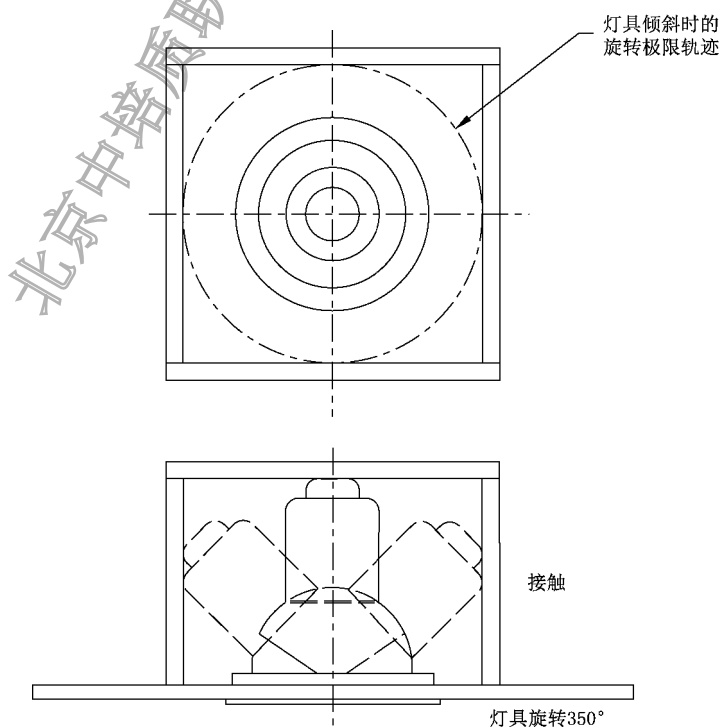
图 D.3 可设置灯具和可调节灯具正确的试验箱尺寸(隔热顶棚)
